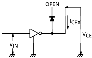
1. I_{CEX}
