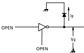
7. V_F
